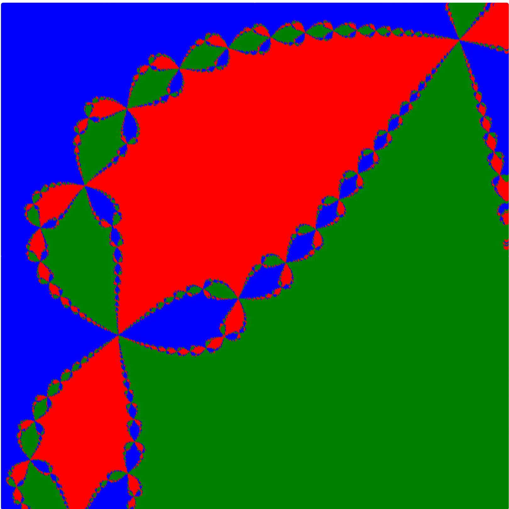
Fractal de Newton (segunda parte)
